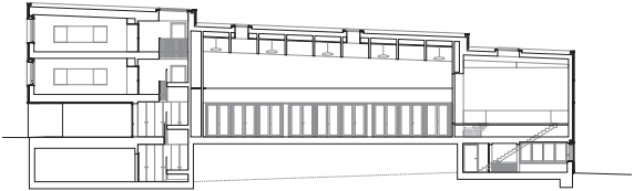
Coupe transversale
